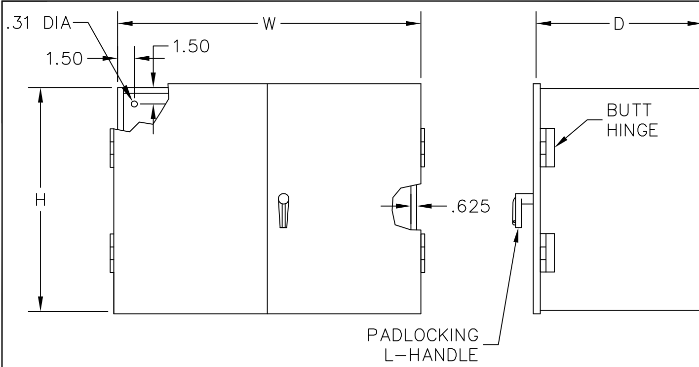
TYPE 1 DOUBLE DOOR CT CABINET
