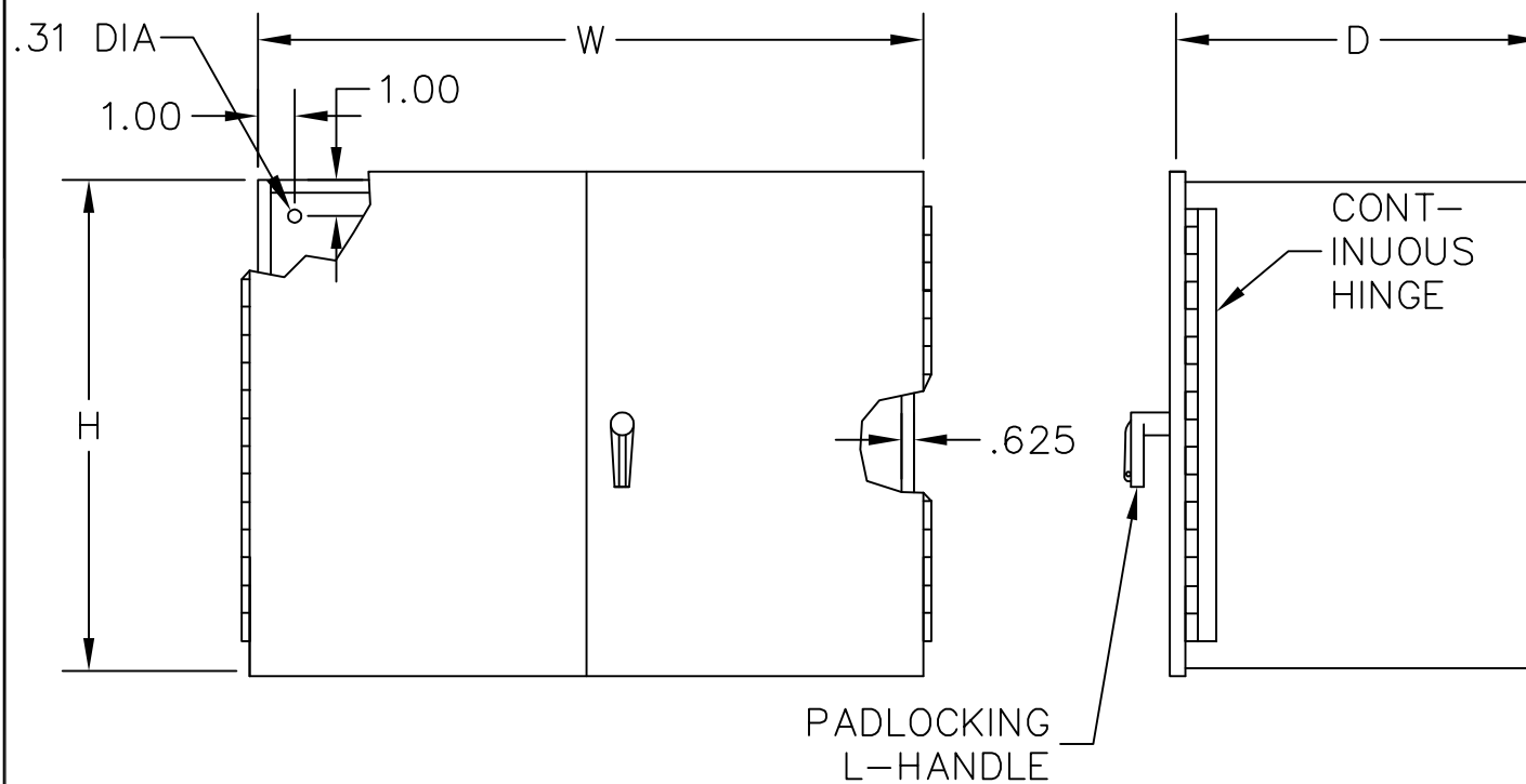
TYPE 1 DOUBLE DOOR CT CABINET
